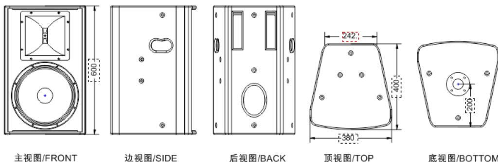
主视图/Front
